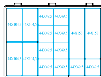
CLASS 32 con 16 vaschette estraibili
